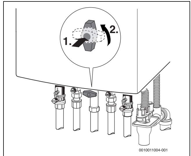
Rys. 5 Otwieranie zaworu gazowego
